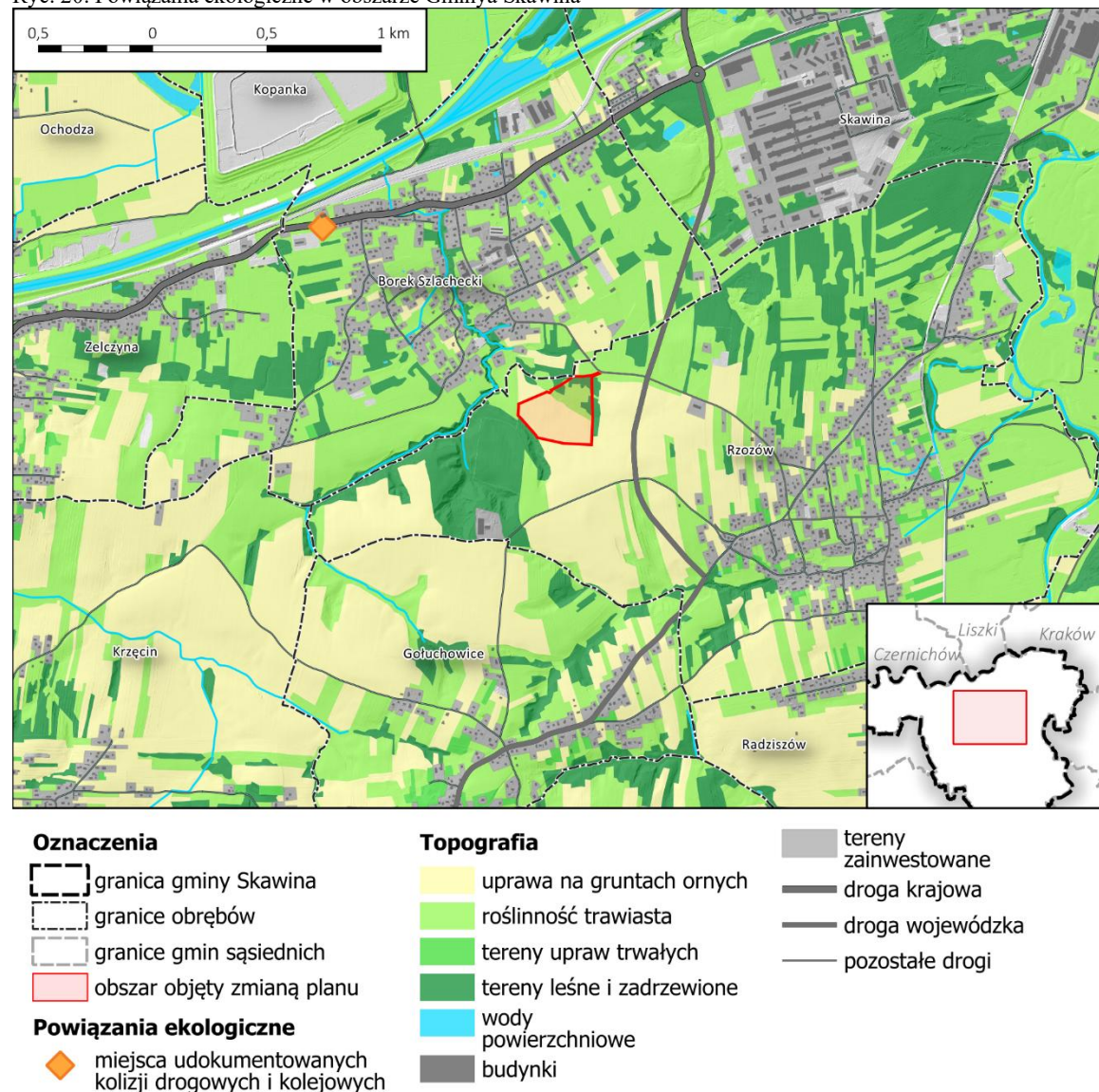
Ryc. 20. Powiązania ekologiczne w obszarze Gminy Skawina
