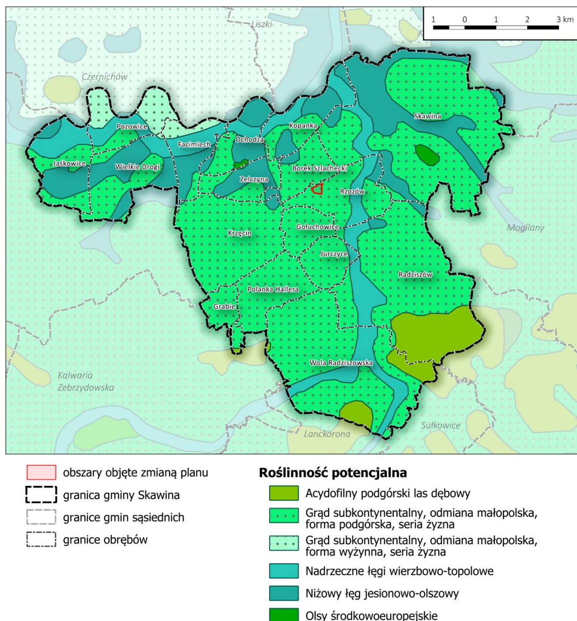
Ryc. 17. Potencjalna roślinność naturalna w Gminie Skawina
