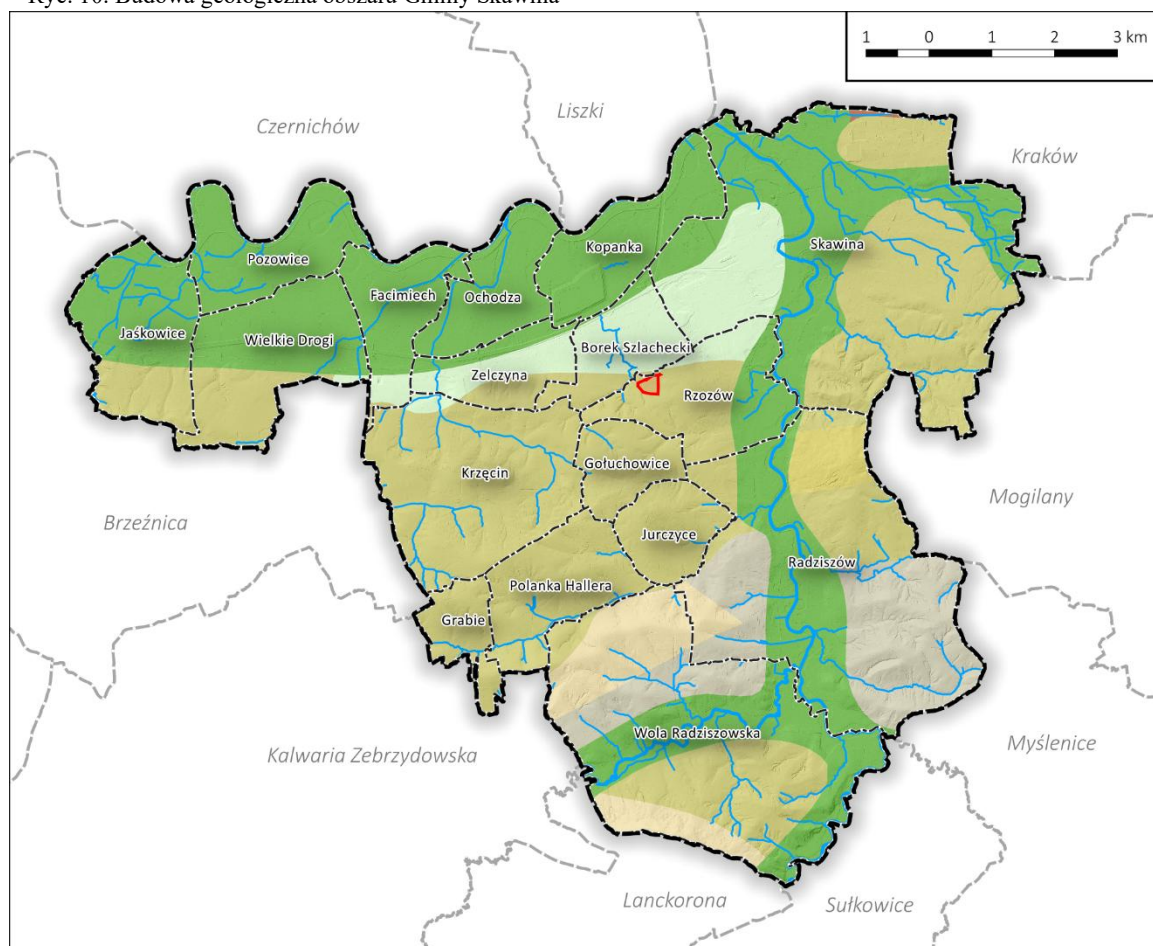
Ryc. 10. Budowa geologiczna obszaru Gminy Skawina
