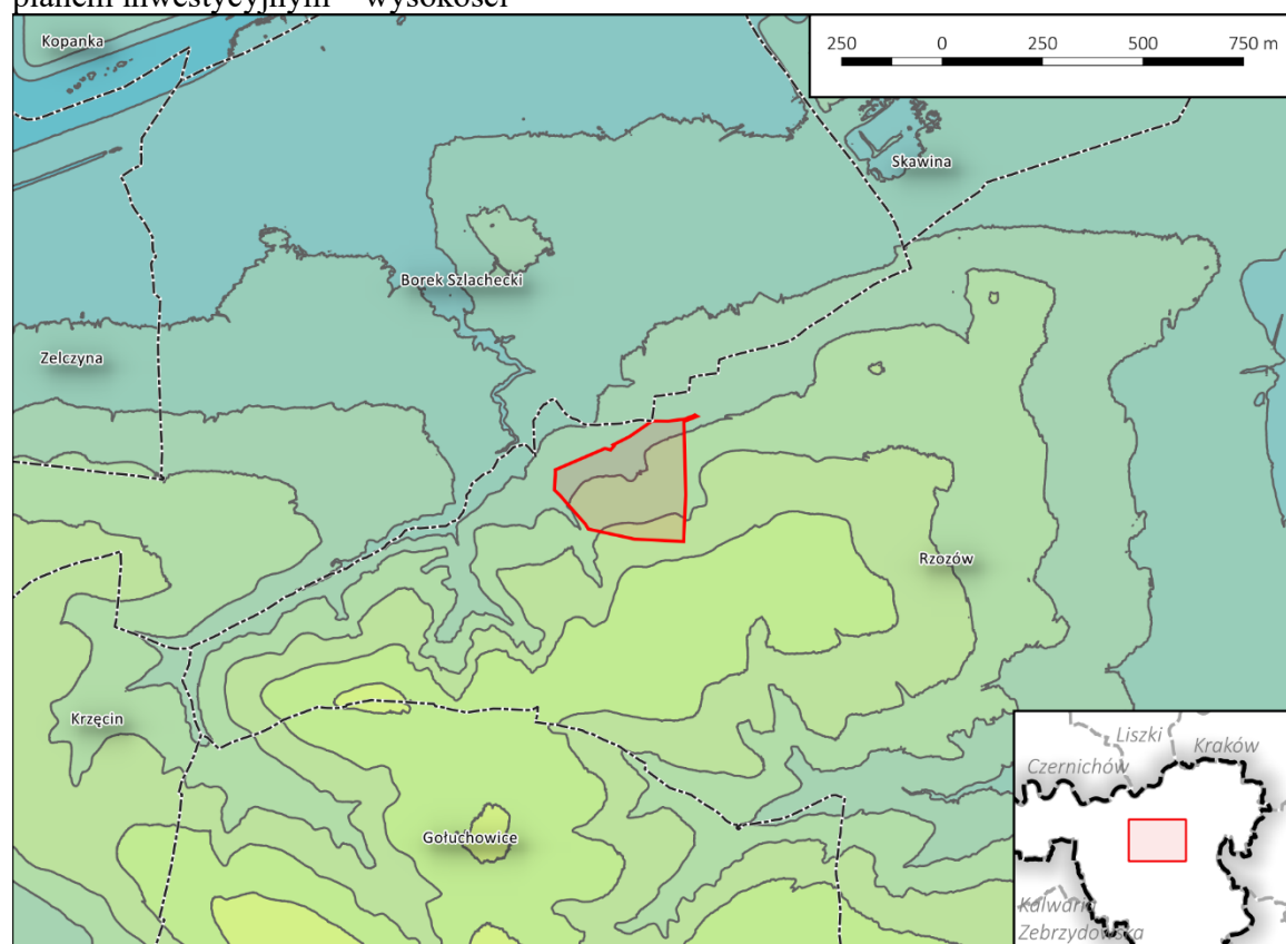
Ryc. 7. Rzeźba terenu Gminy Skawina w sąsiedztwie obszaru objętego zintegrowanym planem inwestycyjnym – wysokości
