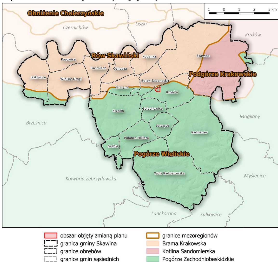
Ryc. 6. Położenie obszaru na tle jednostek fizyczno-geograficznych
