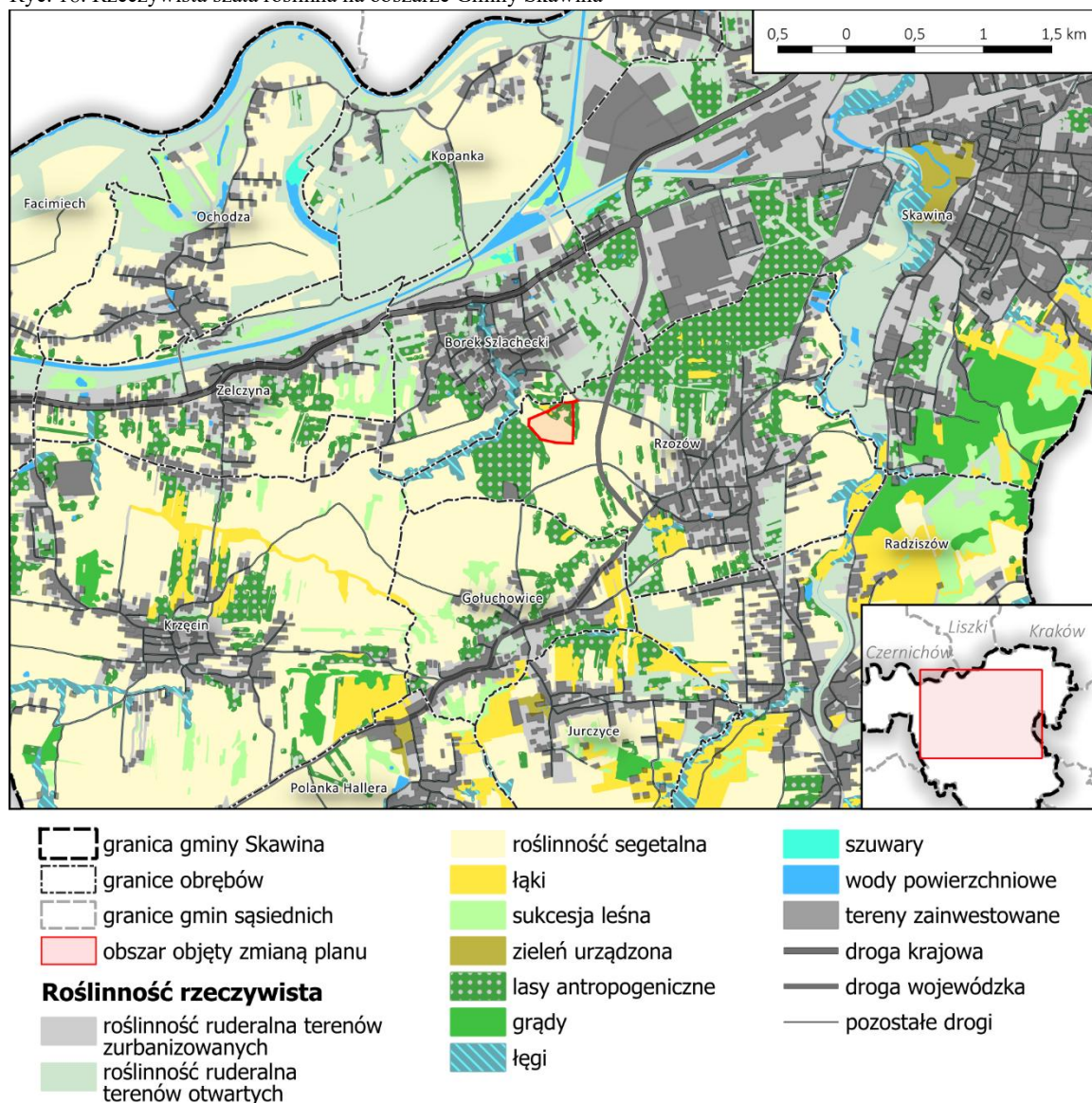
Ryc. 18. Rzeczywista szata roślinna na obszarze Gminy Skawina
