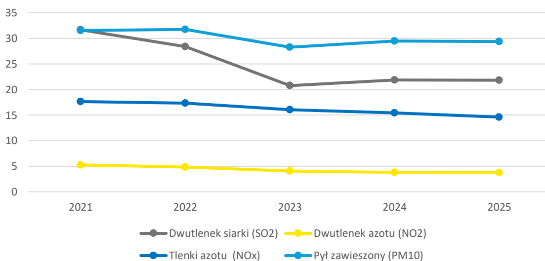
Ryc. 26. Wykres średnich stężeń badanych zanieczyszczeń w Gminie Skawina w latach 2021-2025
