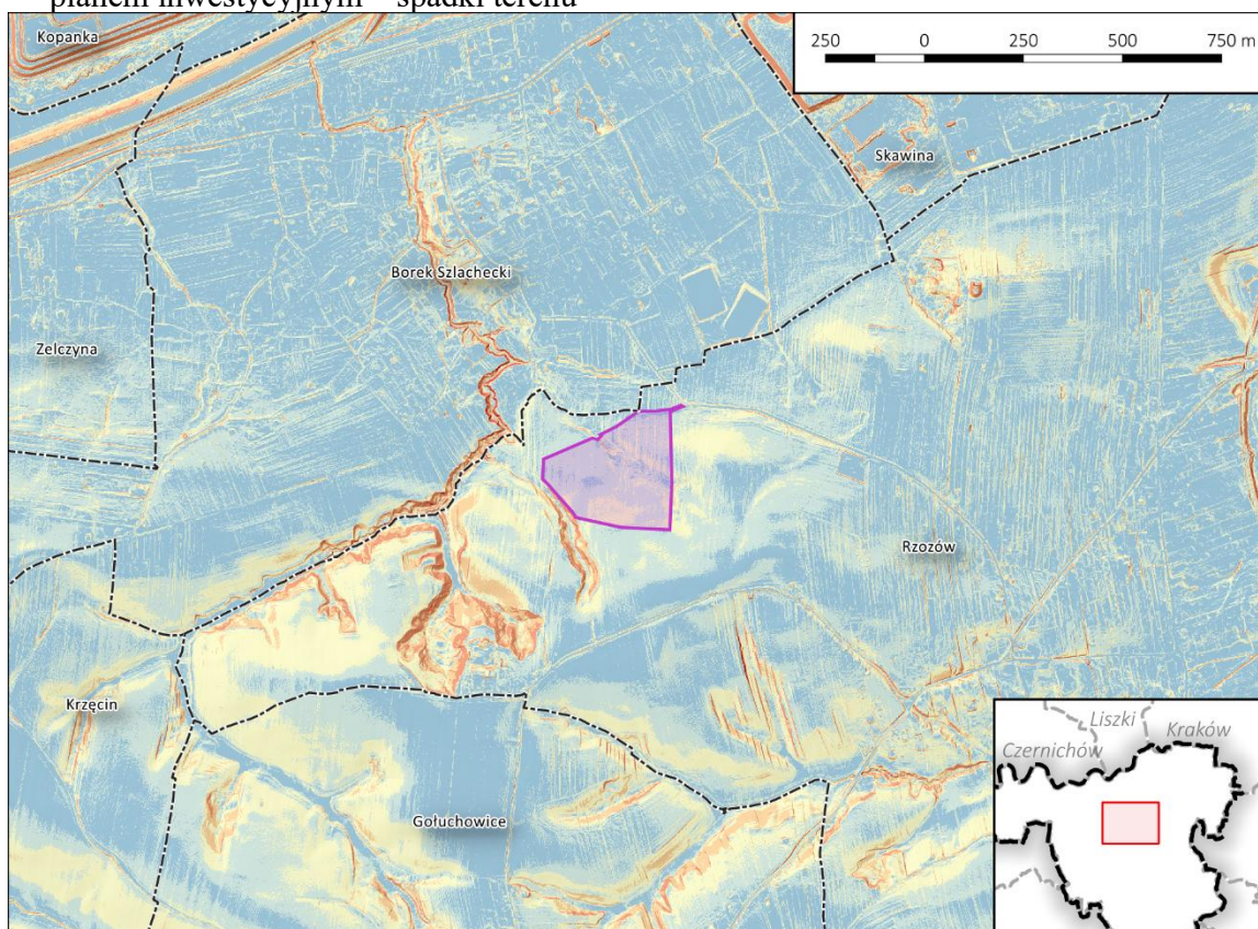
Ryc. 8. Rzeźba terenu Gminy Skawina w sąsiedztwie obszaru objętego zintegrowanym planem inwestycyjnym – spadki terenu
