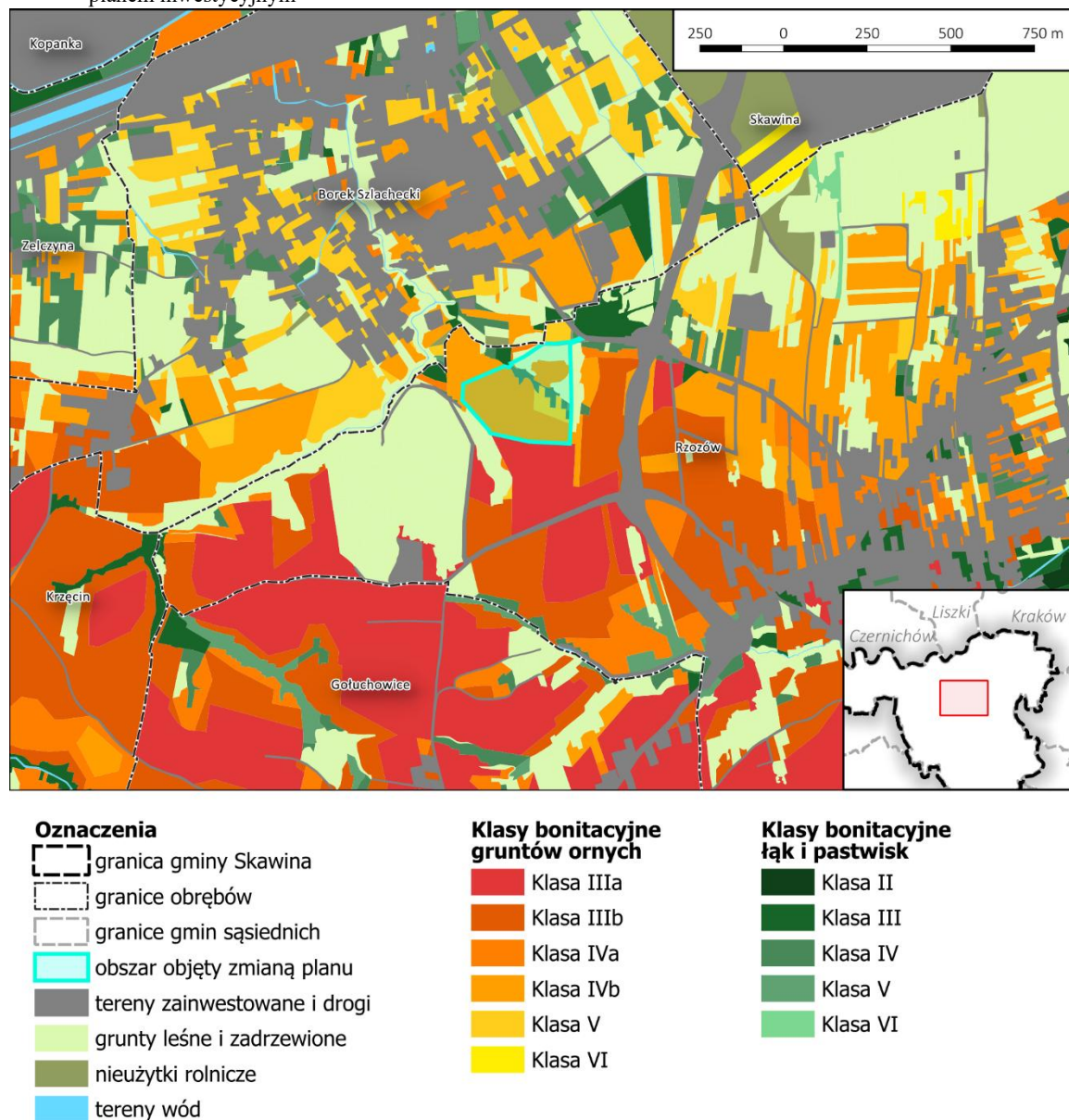
Ryc. 14. Klasy bonitacyjne gruntów rolnych na obszarze miasta Skawina w sąsiedztwie obszaru objętego zintegrowanym planem inwestycyjnym
