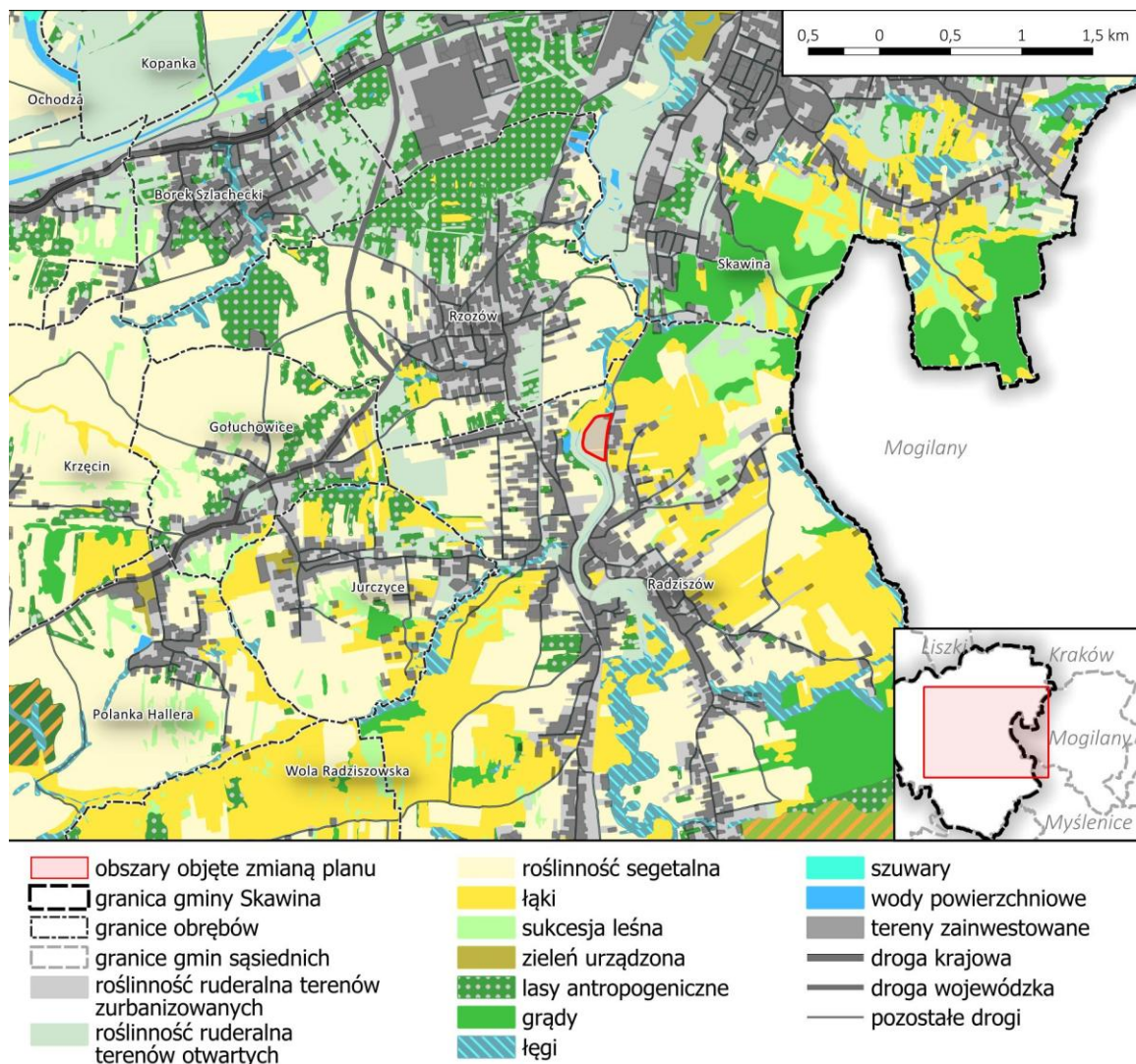
Ryc. 17. Rzeczywista szata roślinna na obszarze północnego Radziszowa i obrębów sąsiednich
