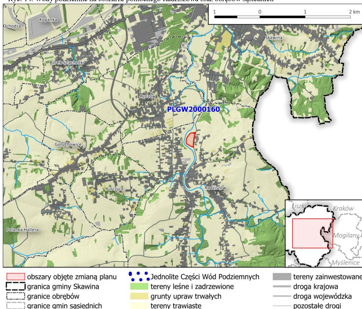
Ryc. 14. Wody podziemne na obszarze północnego Radziszowa oraz obrębów sąsiednich
