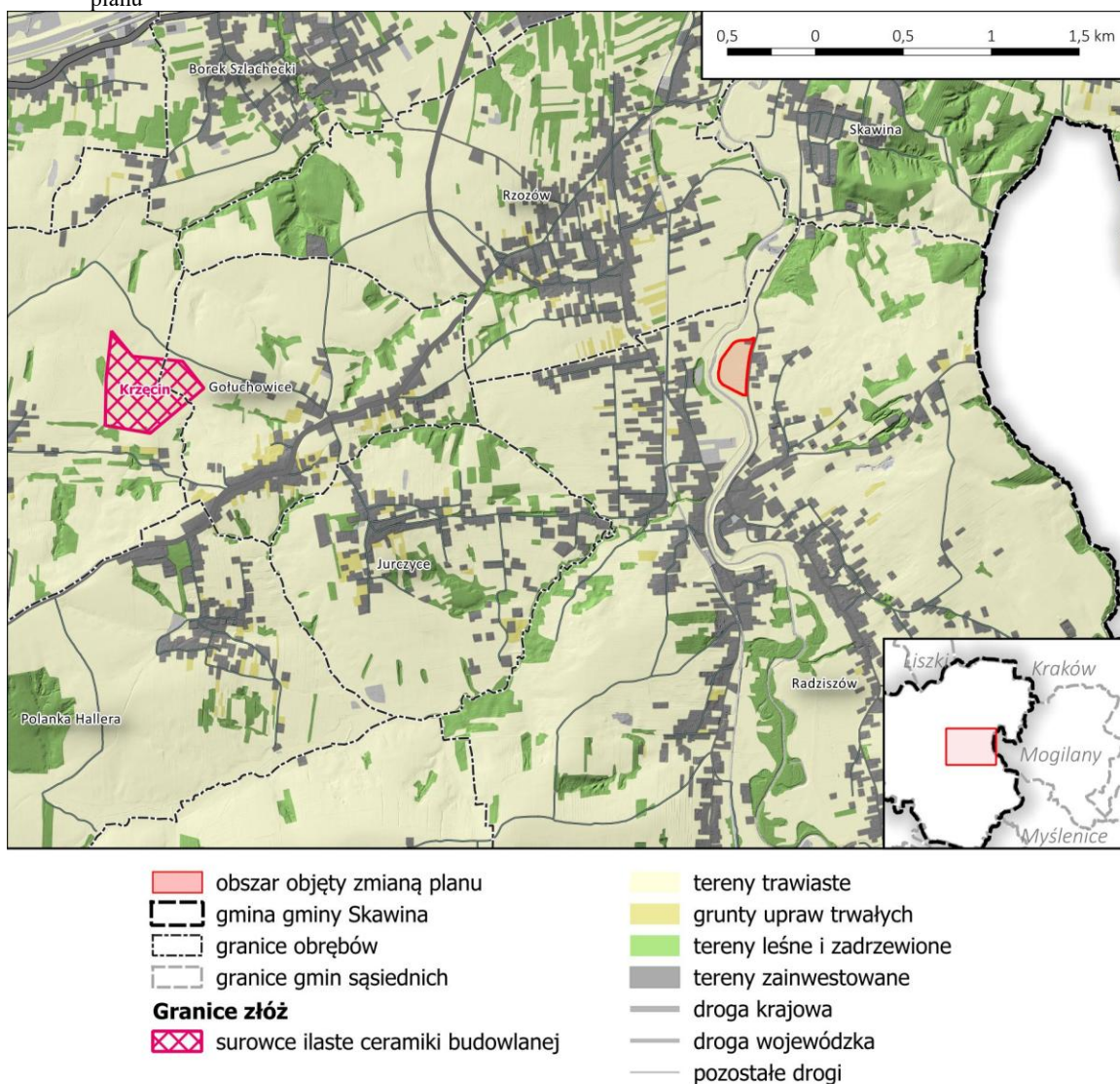
Ryc. 10. Złoża kopalin, obszary i tereny górnicze na obszarze miasta Skawina w sąsiedztwie obszaru objętego zmianą planu
