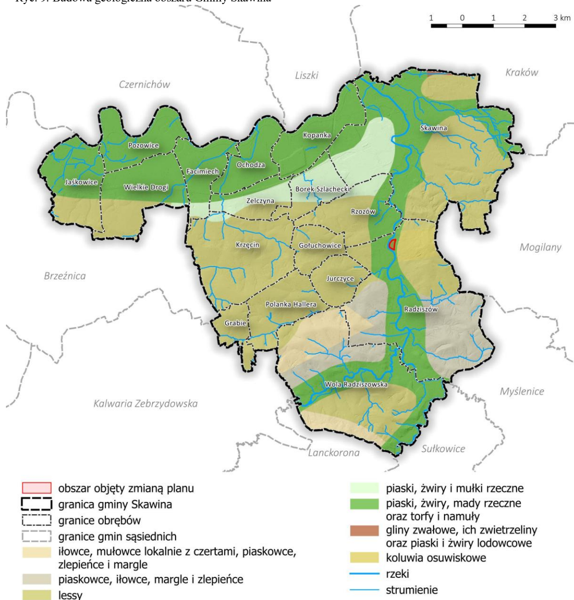
Ryc. 9. Budowa geologiczna obszaru Gminy Skawina
