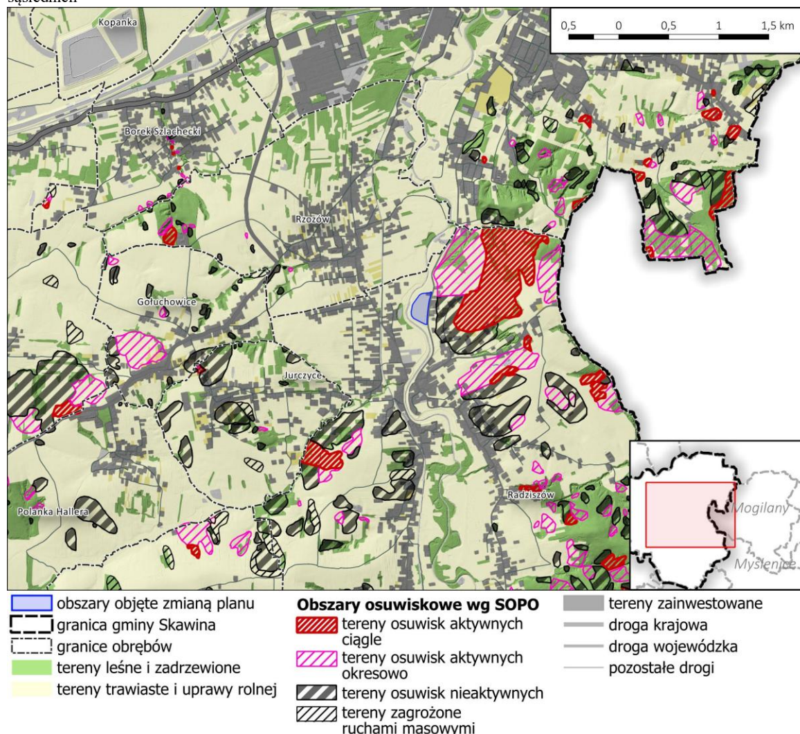
Ryc. 21. Osuwiska i obszary zagrożone ruchami masowymi w obszarze północnego Radziszowa i obrębów sąsiednich
