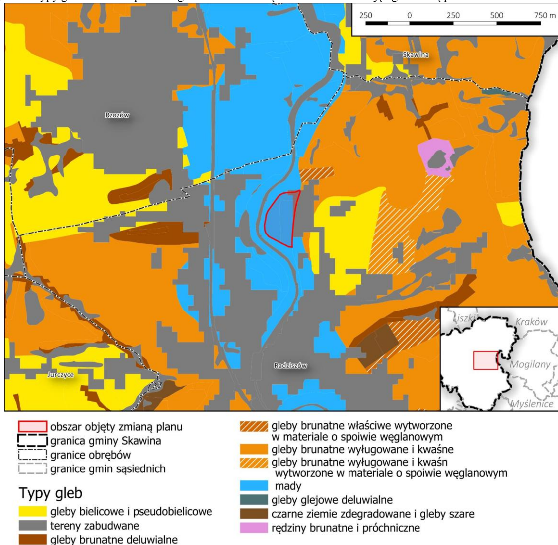
Ryc. 11. Typy gleb na terenie północnego Radziszowa w sąsiedztwie obszaru objętego zmianą planu
