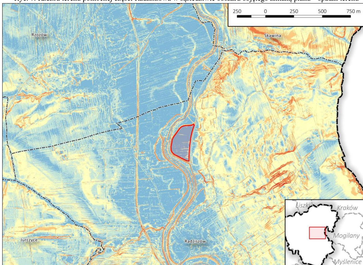
Ryc. 7. Rzeźba terenu północnej części Radziszowa w sąsiedztwie obszaru objętego zmianą planu – spadki terenu
